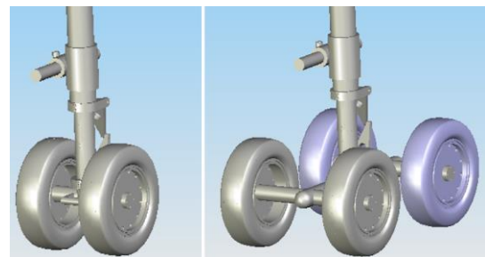
Figure 2 : Atterrisseur simplifié LAGOON : configurations à 2 (gauche) et 4 (droite) roues
