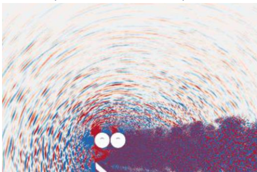
Figure 3 : Simulation numérique par méthode LBM du bruit rayonné par un atterrisseur principal réaliste à 4 roues. Plans vertical (gauche) et horizontal (droite). [2]
